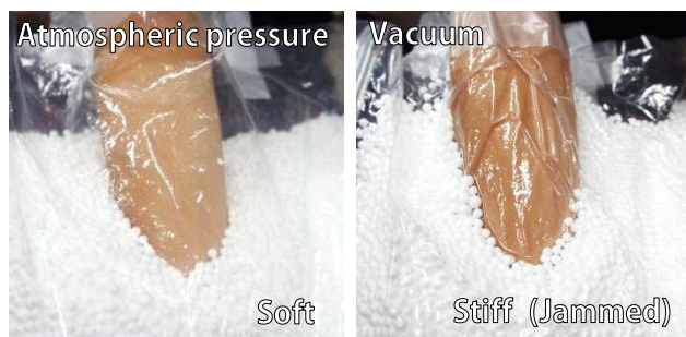
図 2 減圧によるビーズの硬化 Figure 2 Particle jamming by evacuating the air.
