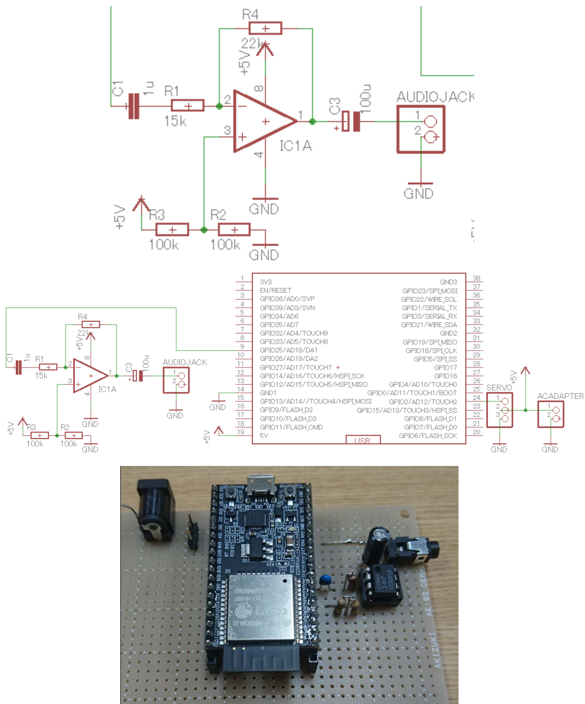
図 9 アナログ出力とオペアンプ回路
