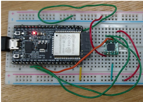
図 4 加速度センサ回路とソースサンプル (※20180220 追記 : GPIO0 は別のポートに変更. http://esp-idf.readthedocs.io/en/latest/api-reference/peripherals/adc.html )
