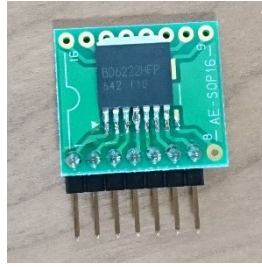
図 16 BD6222HFP のピッチ変換
