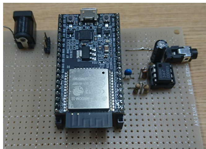
図 8 アナログ出力とオペアンプ回路
