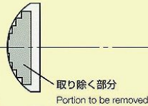
光が直進するレンズ内部 Portion of a conventional convergent lens where rays travel straight
