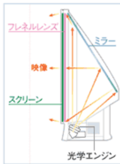
<「HD-61/52MD60」の構造図>
