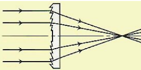
フレネルレンズの光路図 Figure of rays passing through a Fresnel convergent lens
