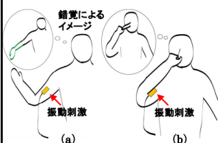
図2 腱振動刺激による運動錯覚 (a) 伸展錯覚, (b) ピノキオ錯覚
