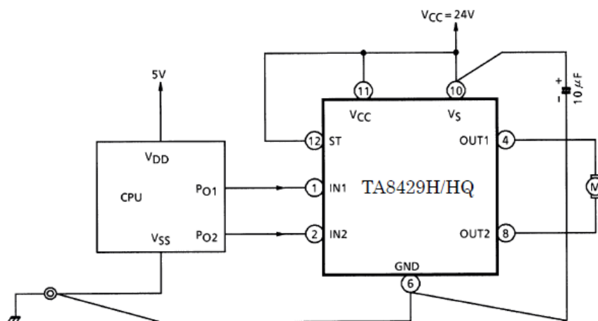
図 10 駆動回路(TA8429 マニュアルより)
