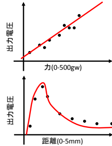
フォトトリフレクタを用いた近接距離センサ
