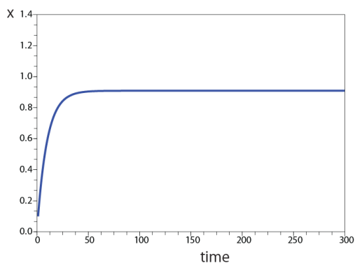
PD制御 : P=10, D=10
