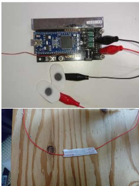
図 1 開発した機械刺激装置
