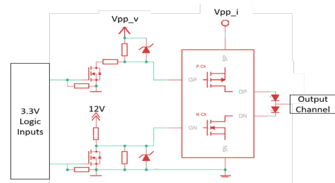
図 3: スwitchングに用いる Half Bridge 回路。P MOS FET ののゲート電圧をプルアップする電源 (Vpp_v) は Vpp_i から高耐圧 NMOSFET を用いたソースフォロワによって生成。またハーフブリッジの入力電圧が 10V 程度に収まるようにツェナーダイオードを入れている。
