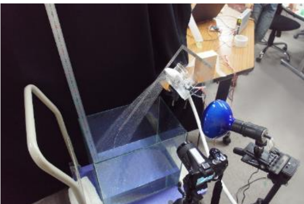
図 5 実験風景
