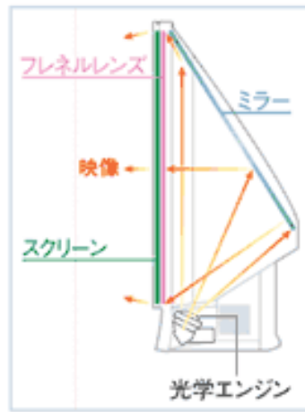
<「HD-61/52MD60」の構造図>
