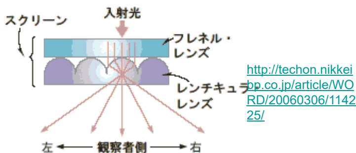
<「HD-61/52MD60」の構造図>
