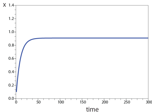
PD制御 : P=10, D=10
