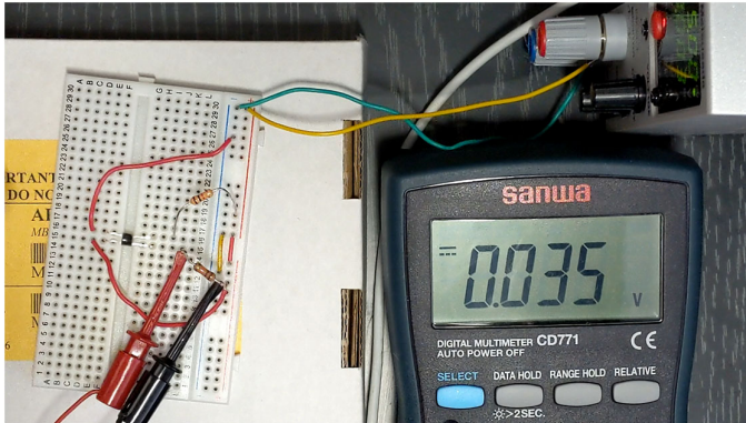
フォトリフレクタを用いた近接距離センサ
