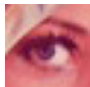
Bi-Linear法
